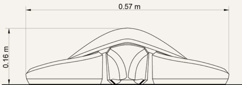
VISTA LATERAL
